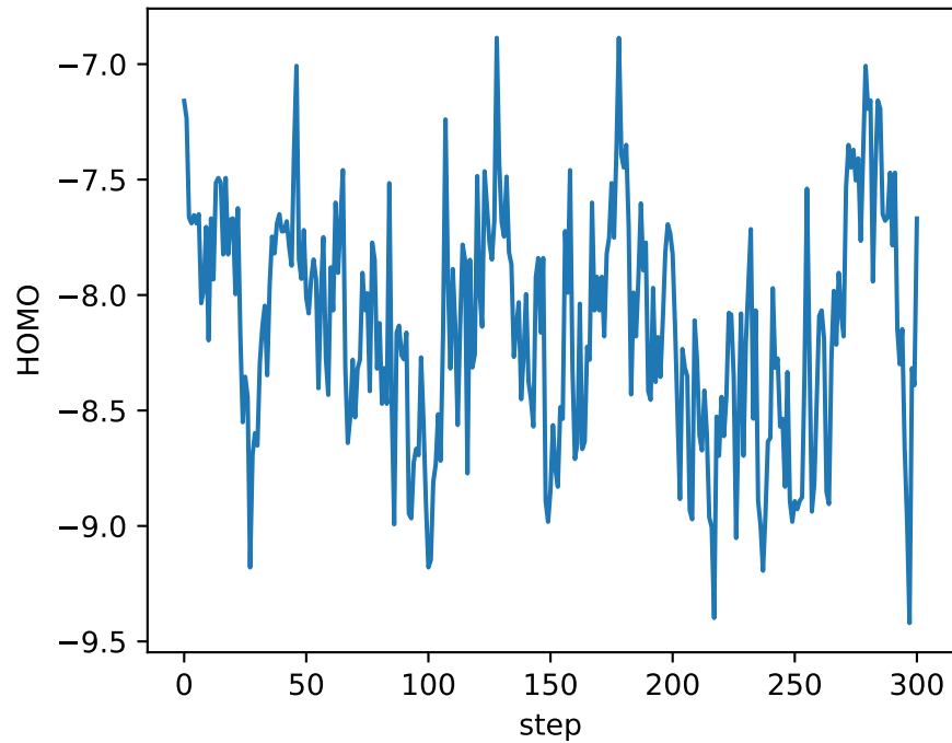
HOMO - evolution
