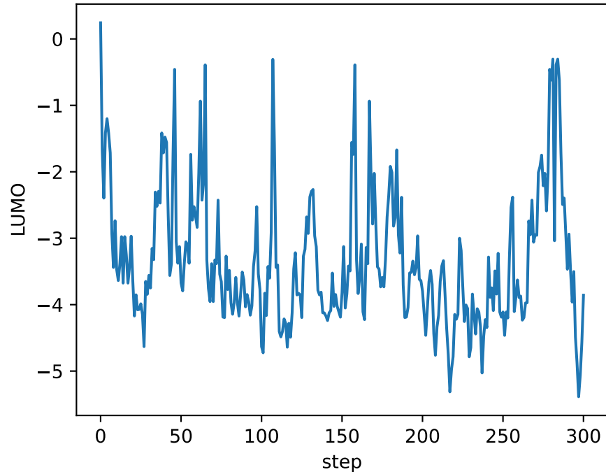
LUMO - evolution
